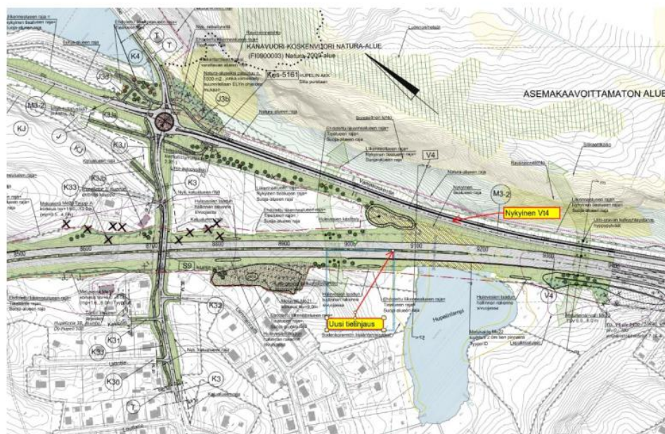
Kuva 6-2. Vt4 Tiesuunnitelman ympäristösuunnitelmakartta paaluvälillä 8500–9400.
